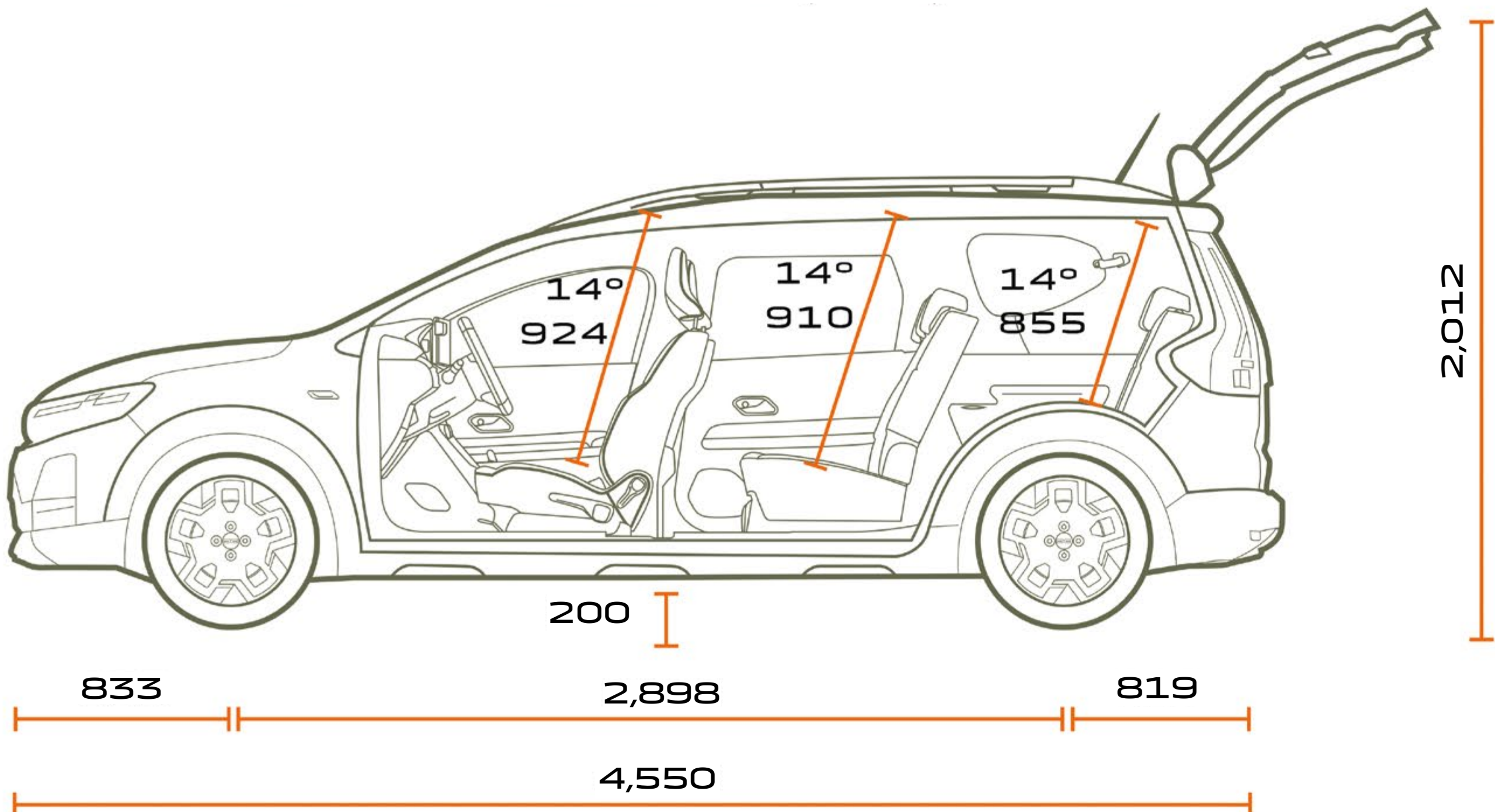
FRÅN SIDAN
