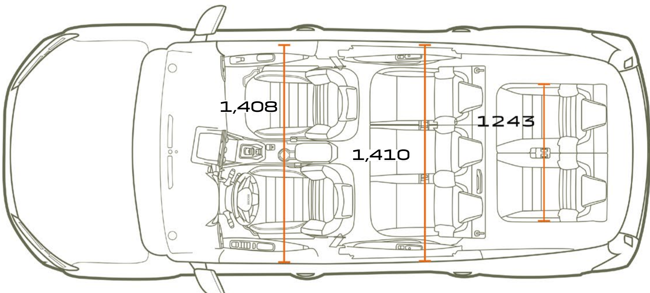
FRÅN OVAN
